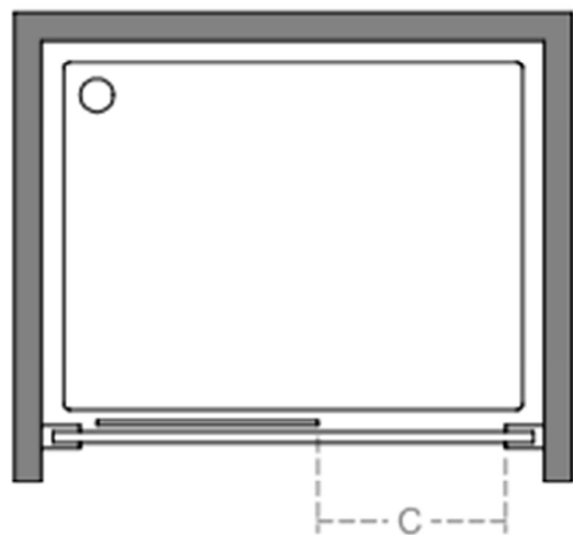
Piatto tra due pareti
