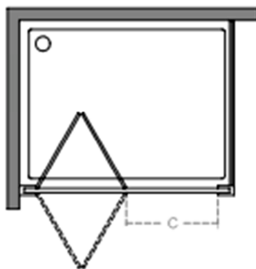
Piatto angolare+fianco
